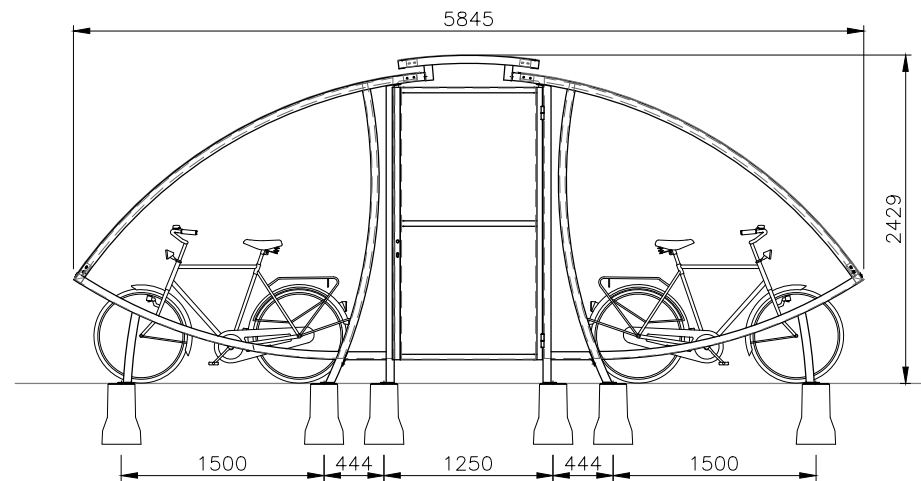
Looppadafsluiting met enkele deur
